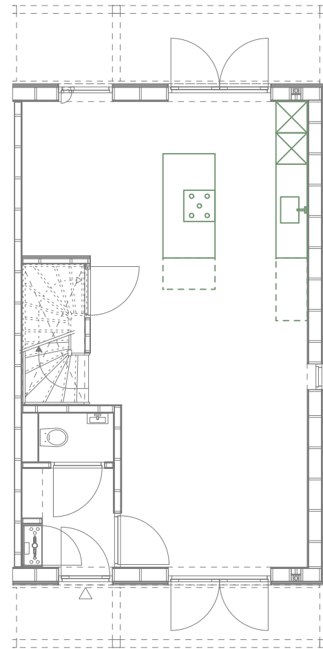
A.03 - keuken positie B (buitengevel noordzijde)
