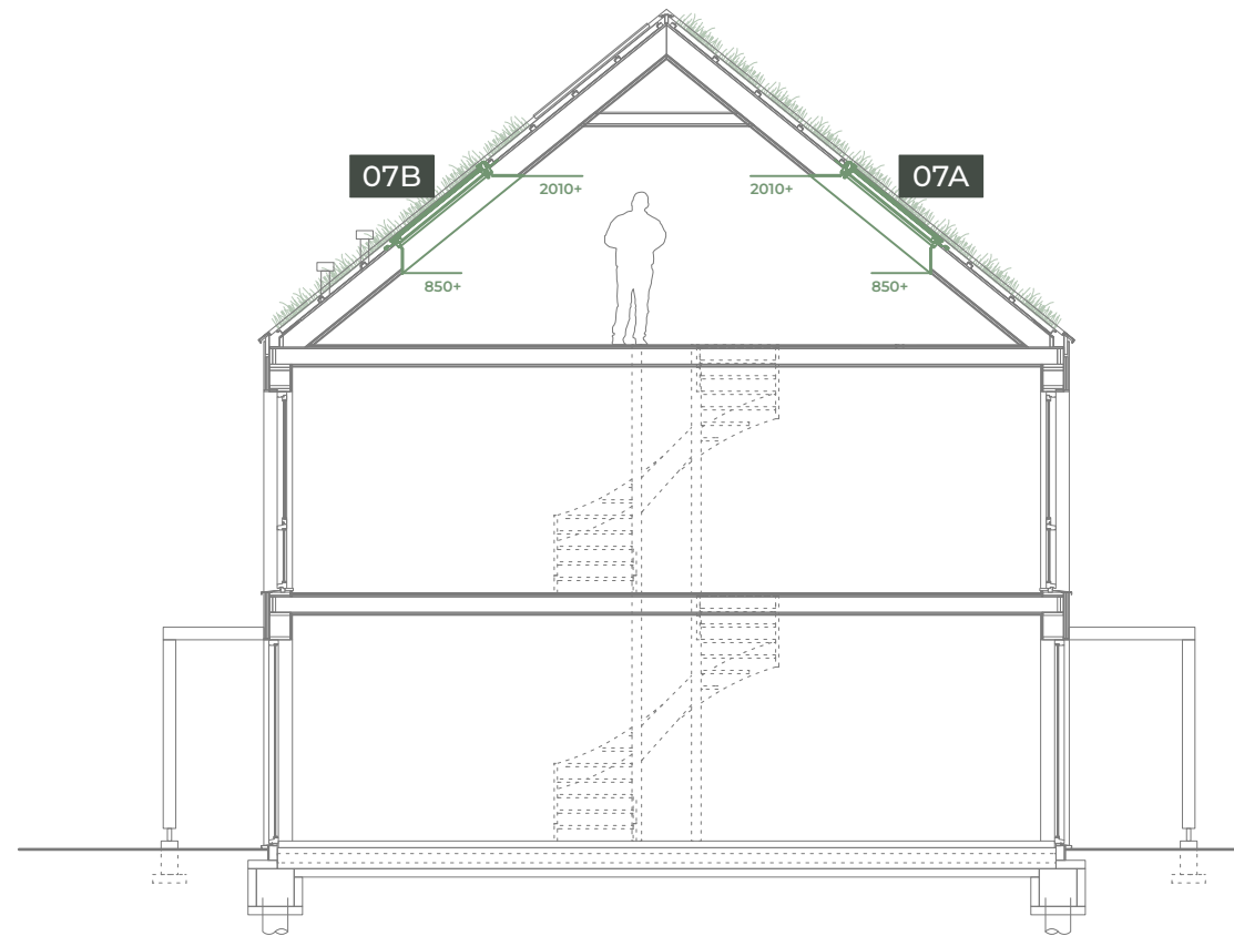
DOORSNEDE
