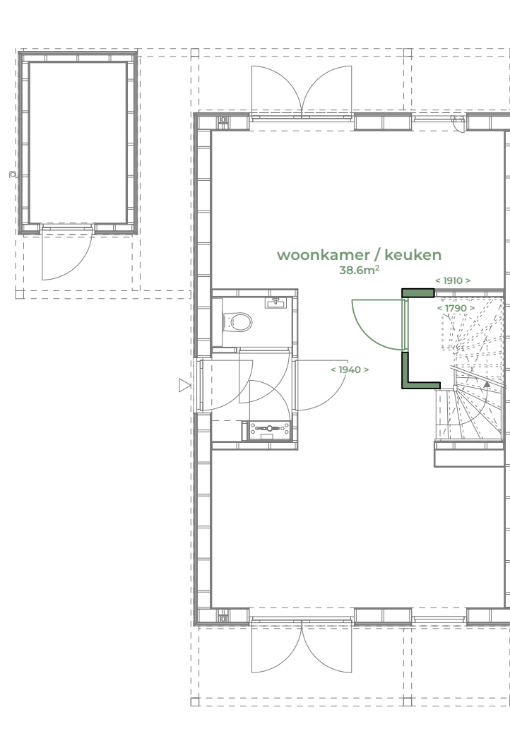
BEGANE GROND
