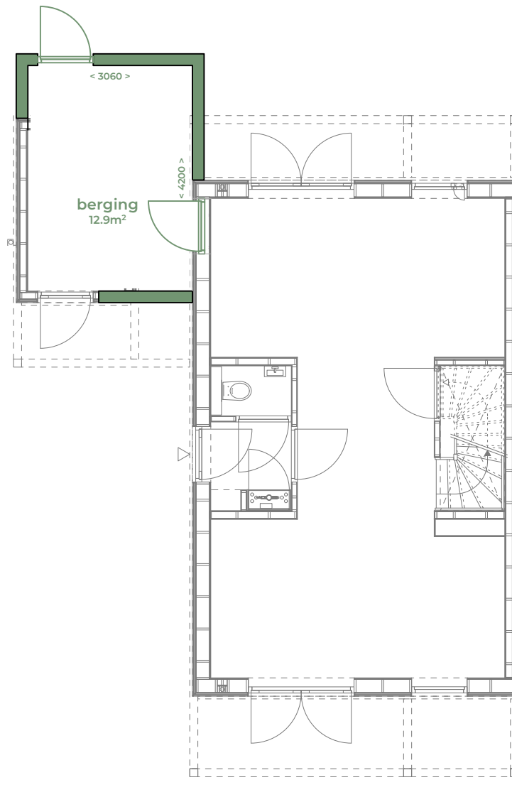
BEGANE GROND
