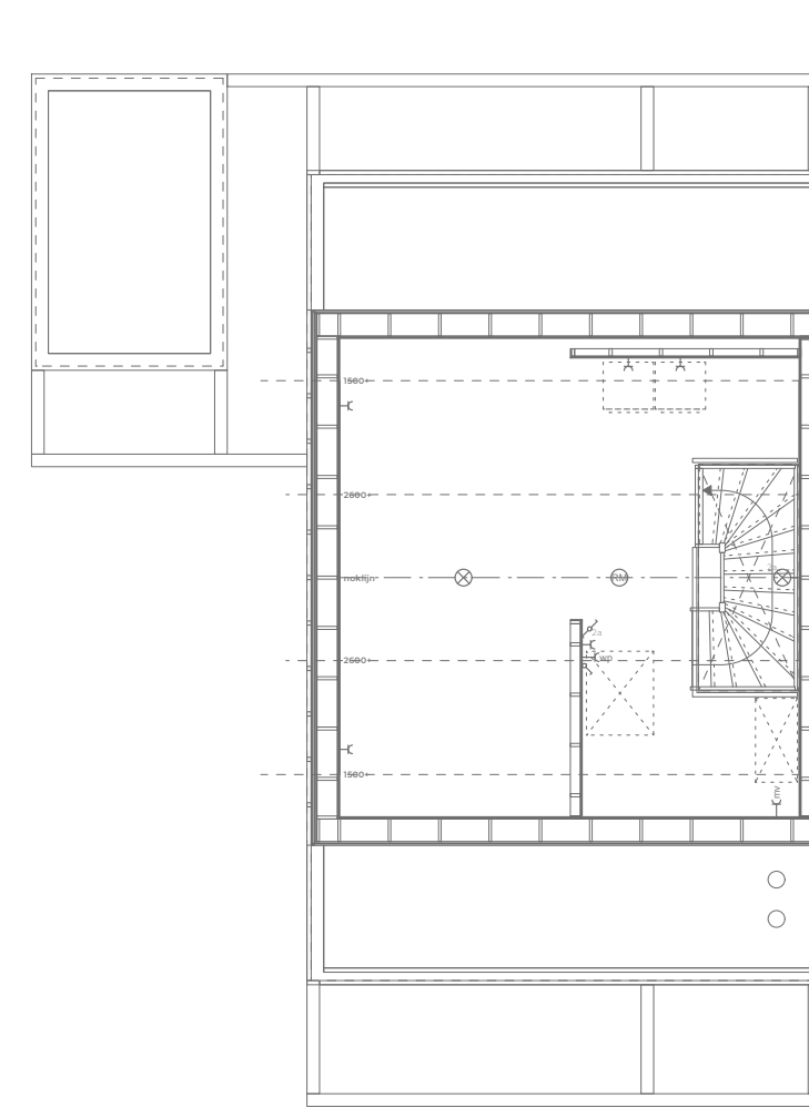
TWEDE VERDIEPING
