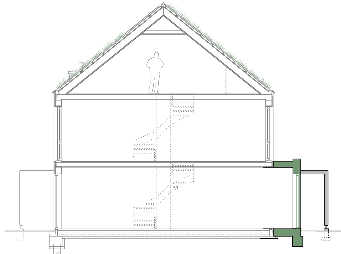
DOORSNEDE
