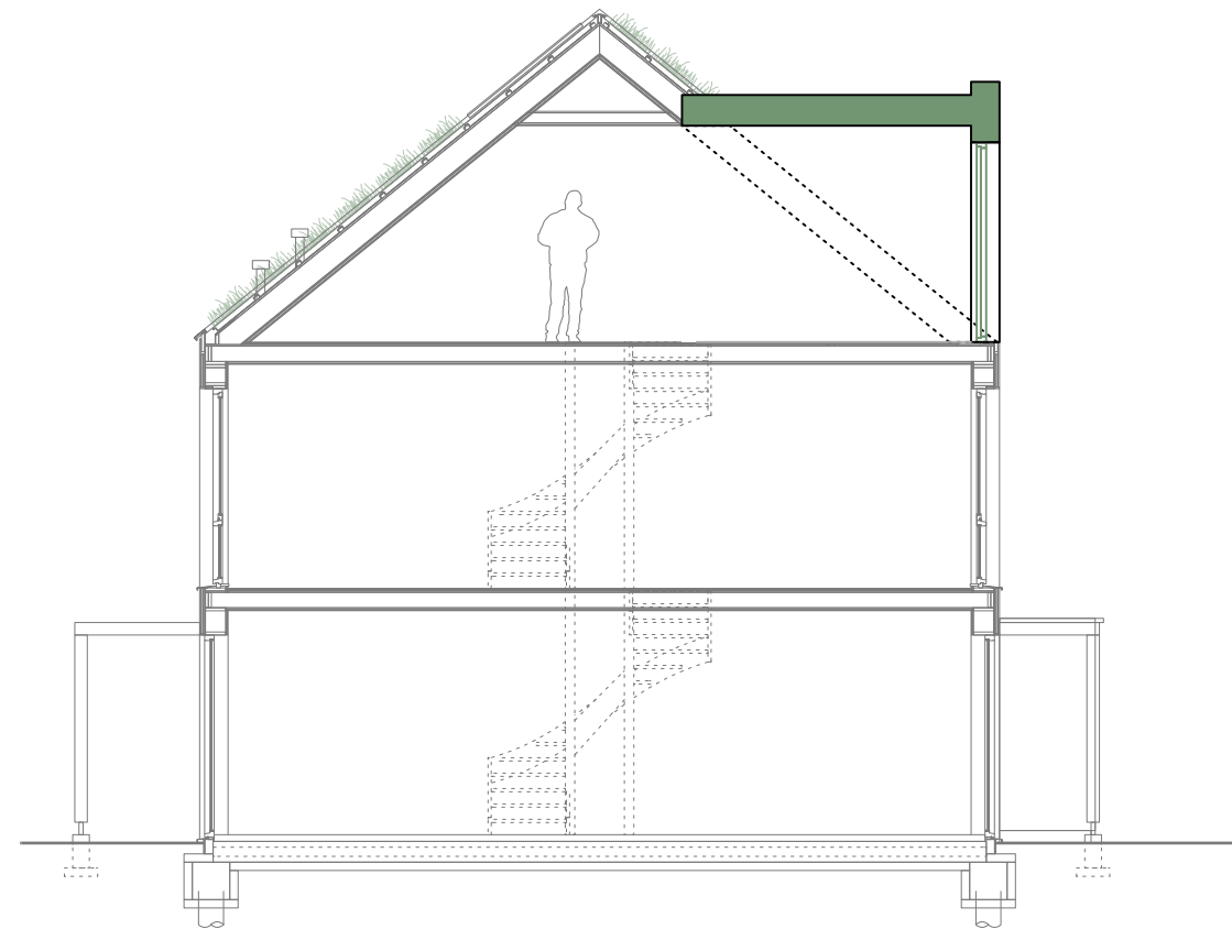
DOORSNEDE
