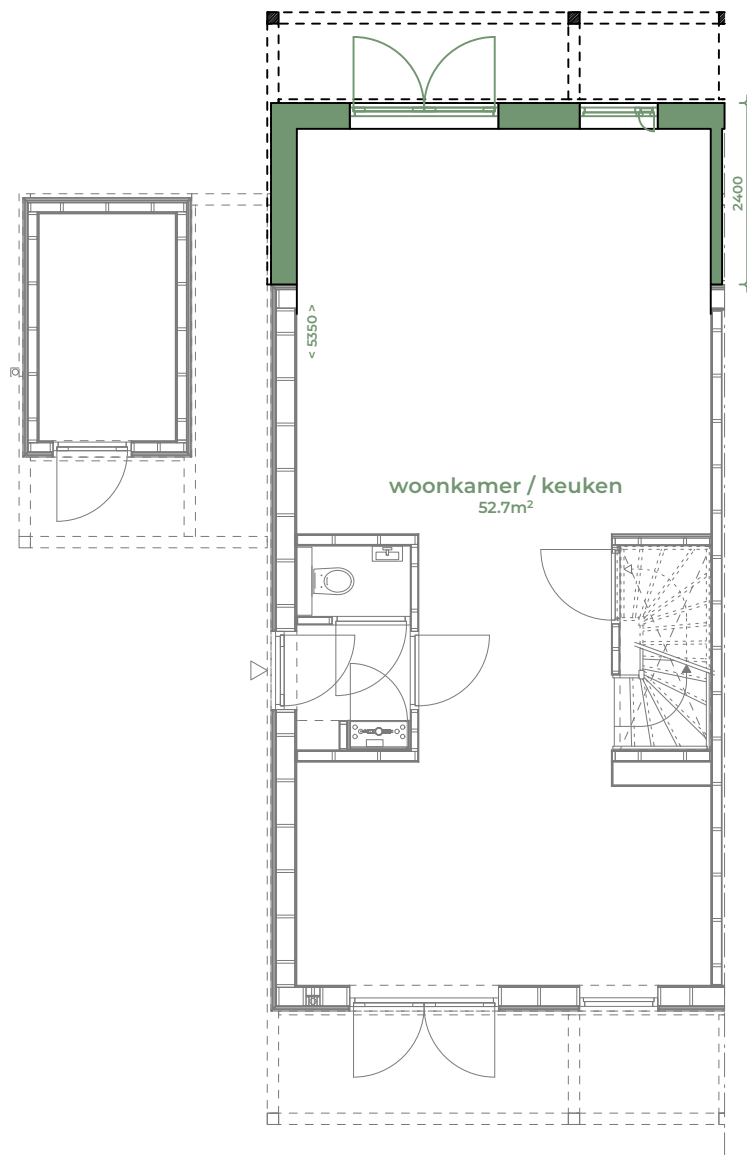
BEGANE GROND
